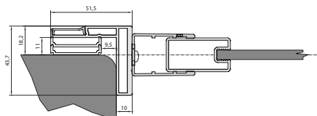
Profil EPB (AN13-ANT1)
