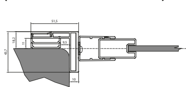
Profil przyścienny EPB (SOLT1-SOLT2-SOL13-SOLF13)
