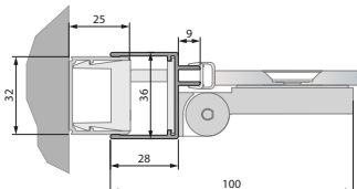
Profil przyścienny 50445 (AN1C)
