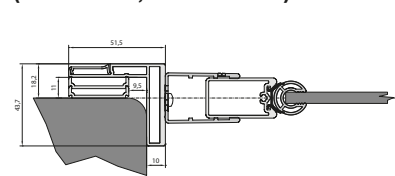
Profil EPB (SOL1-SOL2, SOLF-SOLB2)
