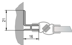
Profil przyścienny domykowy 50418
