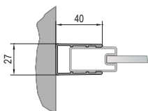
Profil przyścienny 50012 (ANT1, AN13, ANR)
