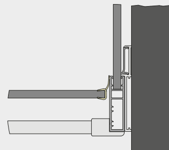
Detal A - widok z góry
