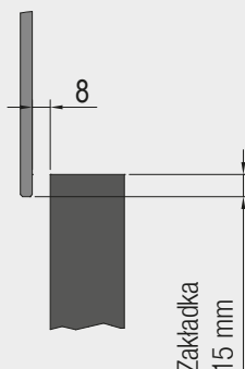
Detal A - widok z przodu
