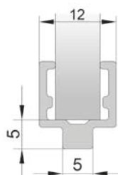
Profil aluminiowy chroniący dolną krawędź szkła i ułatwiający montaż.
