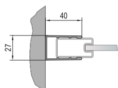
Profil przyścienny 50012
