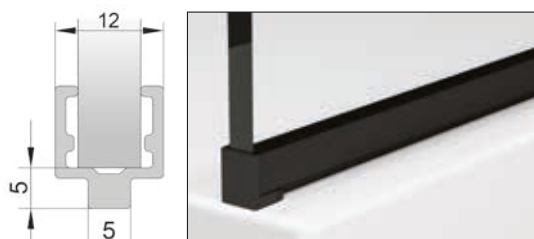
Profil aluminiowy chroniący dolną krawędź szkła i ułatwiający montaż.
