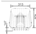
Kosz na naczynia ze stali szlachetnej 507 829
