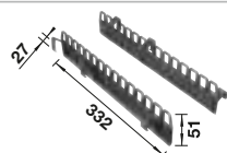
BLANCO SELECT Clip Uchwyt do worka na śmieci 521 300
