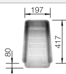
Odsączarka ze stali szlachetnej 227 692
