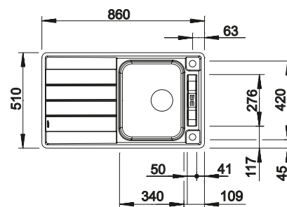
Głębokość komory/komór: 190/40 mm
