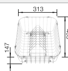
Kosz na naczynia ze stali szlachetnej
