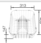
Kosz na naczynia ze stali szlachetnej 507 829
