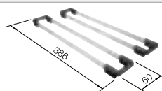
Zestaw szyn ETAGON
